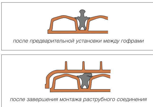
Рис. 2.5 Положение уплотнительной прокладки
