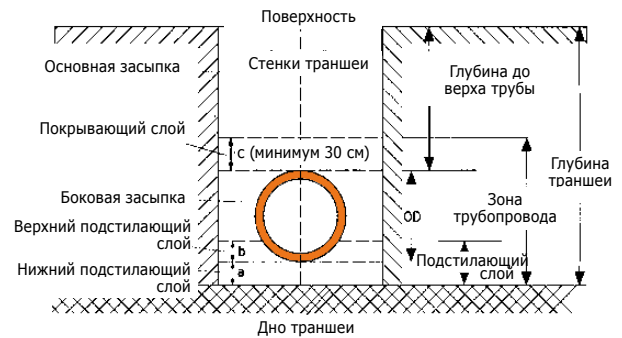
Рис. 3 Устройство траншеи
