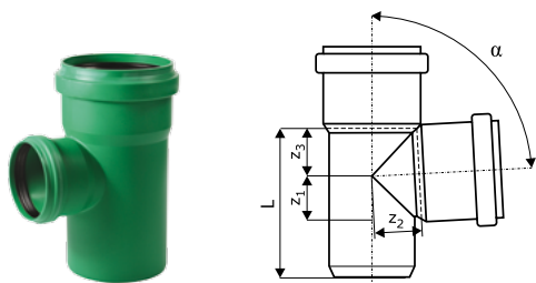
KG2000EA – тройник 87°
